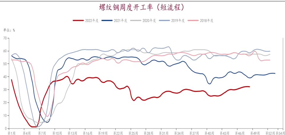
图 7：螺纹钢短流程开工率（单位：%）
