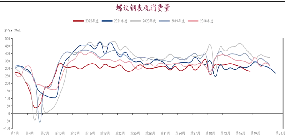
图 8：螺纹钢周度表观消费量（单位：万吨）
